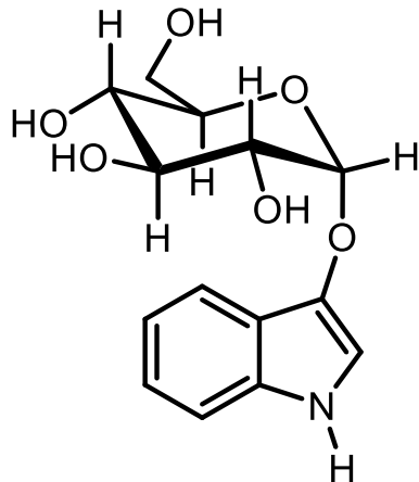
Indican (aus Indigopflanze indigofera tinctoria )
